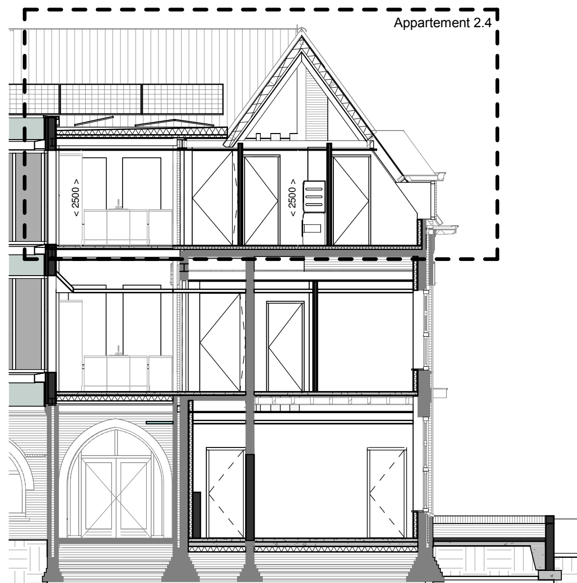
Doorsnede 2.4
