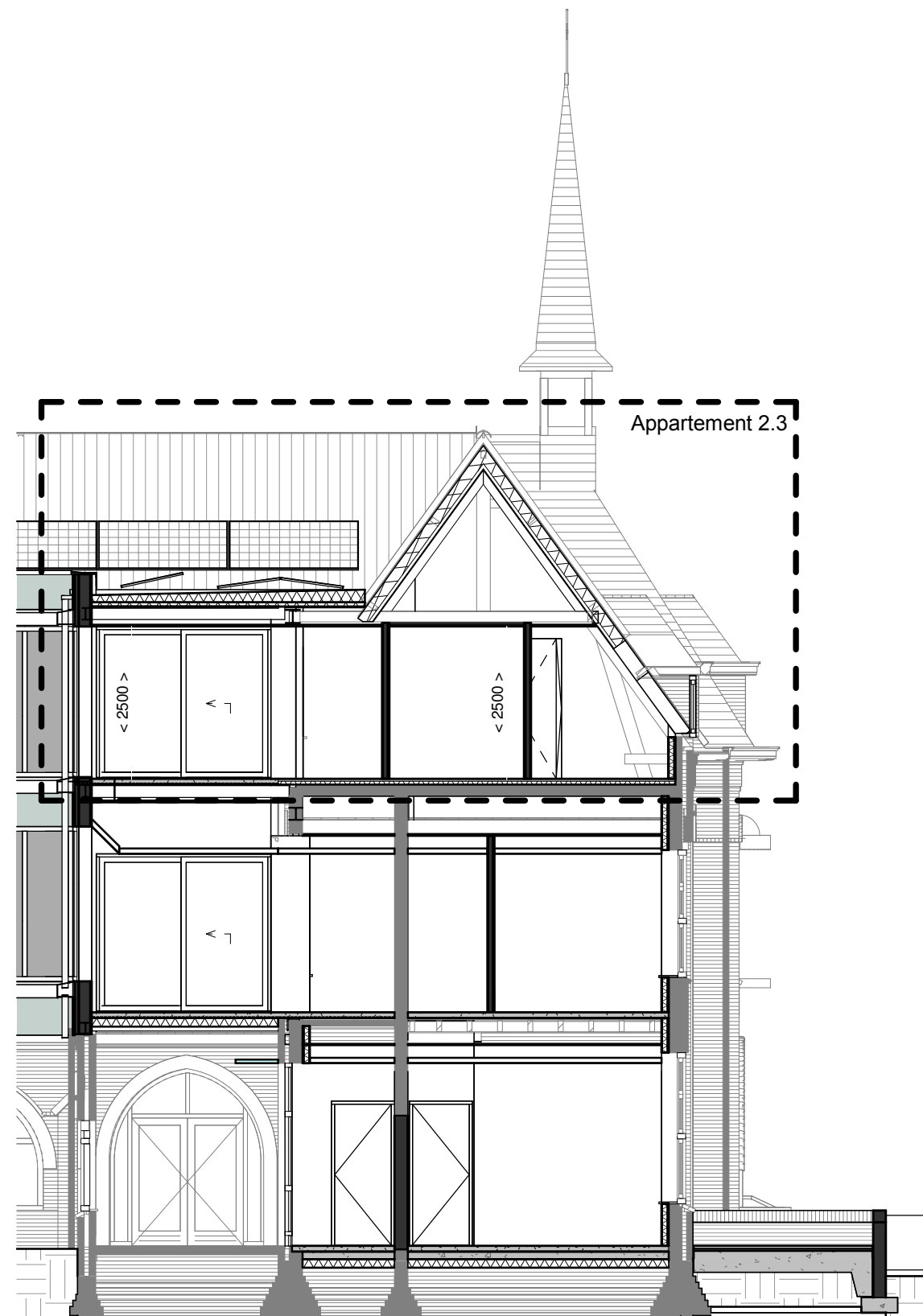
Doorsnede 2.3
