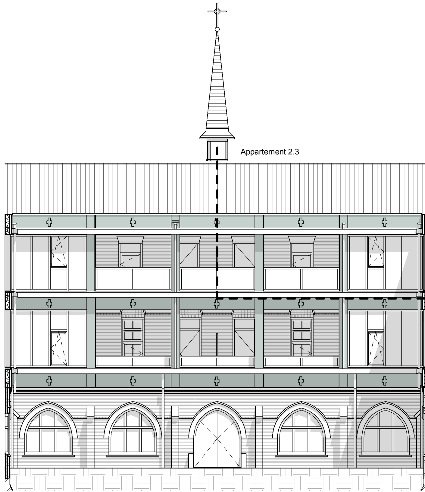
achtergevel
