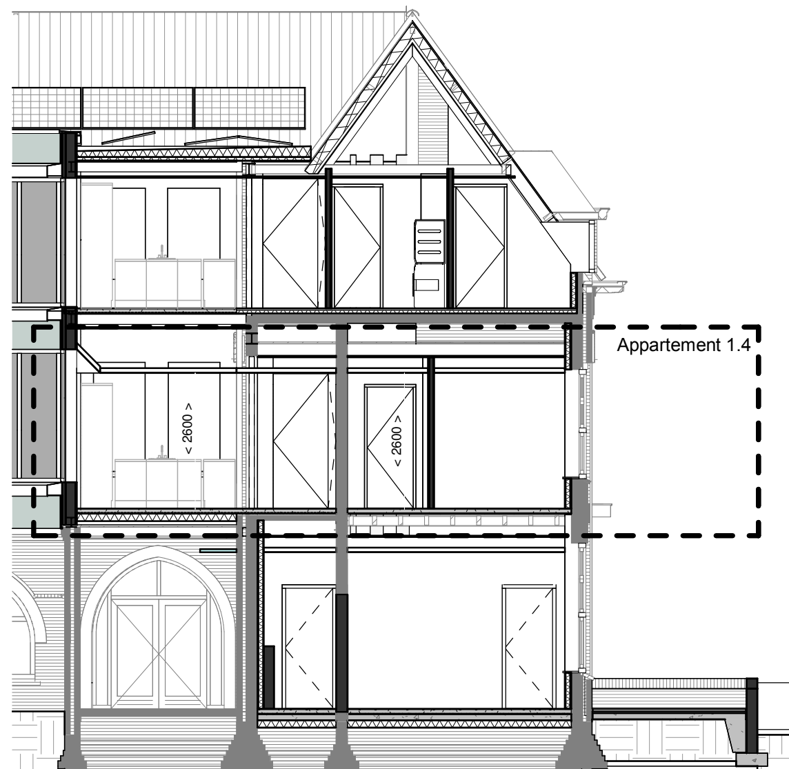
Doorsnede 1.4
