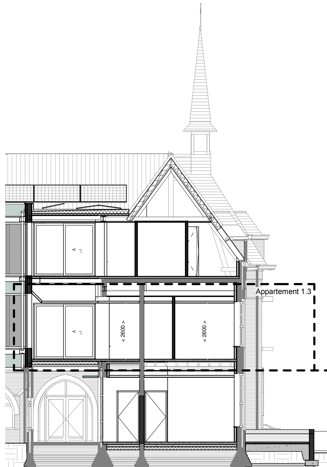
Doorsnede 1.3
