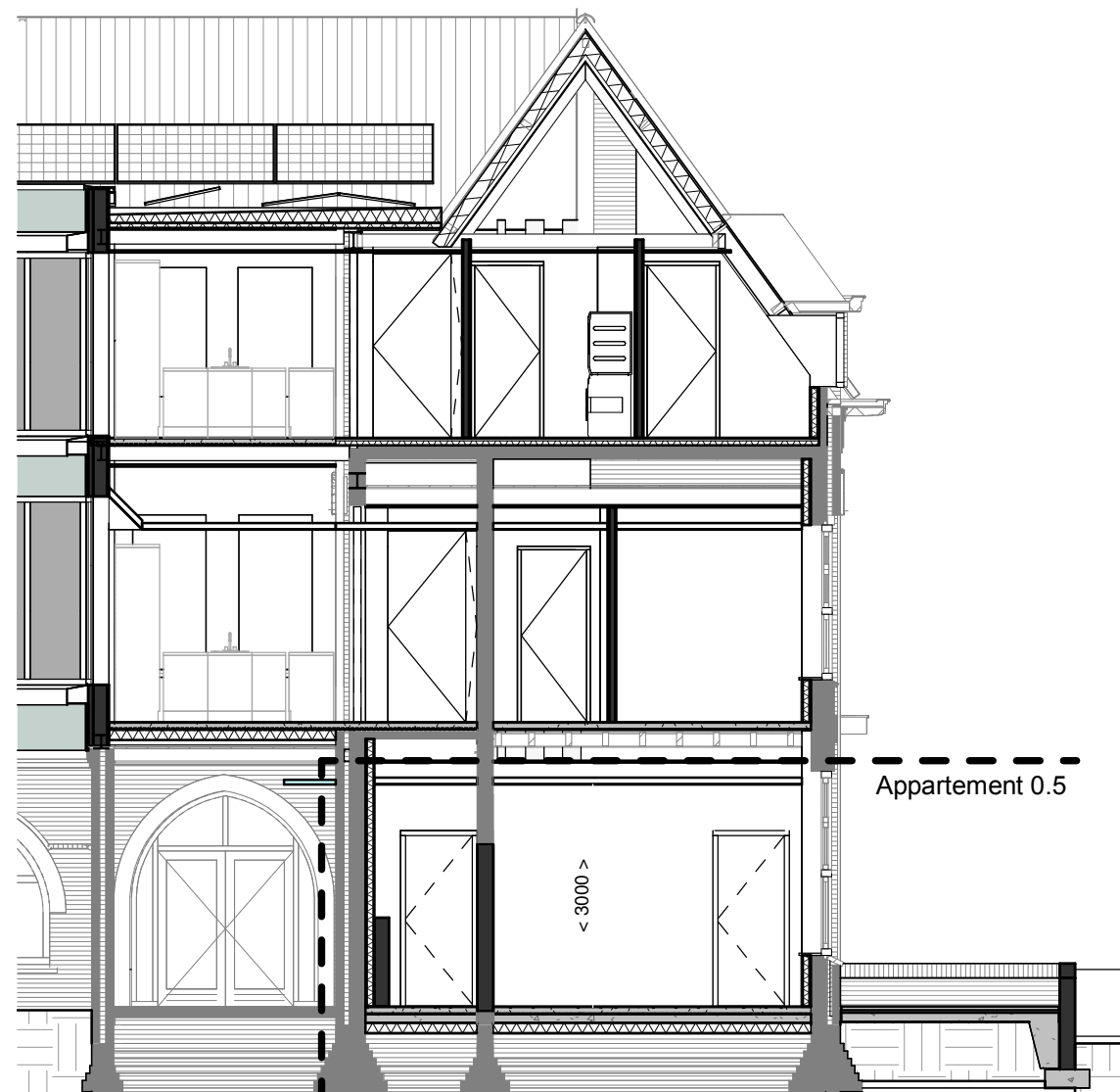
Doorsnede 0.5
