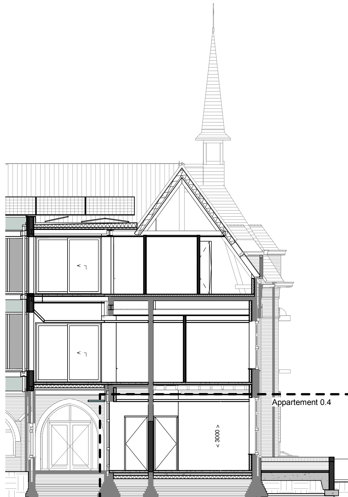
Doorsnede 0.4
